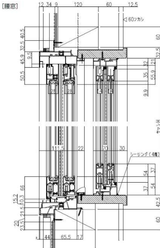
(縦断面)
