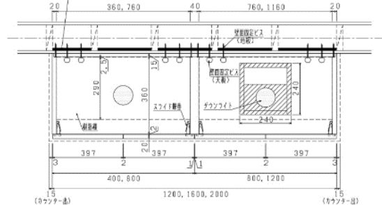
平面詳細図
