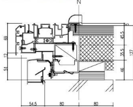
[2 階 FS パルコニー下枠断面]
