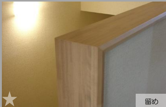
笠木端部納まり (K2笠木)
