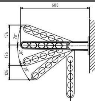
2 階 (ハイウォールバルコニー)
