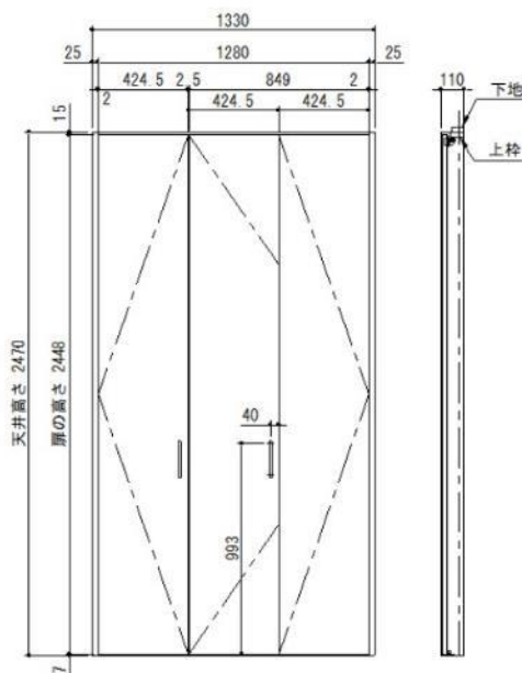
本図は吊元：右を示す
