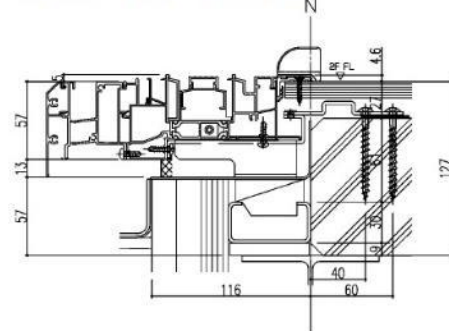
[2 階 2FLF 下枠断面]
