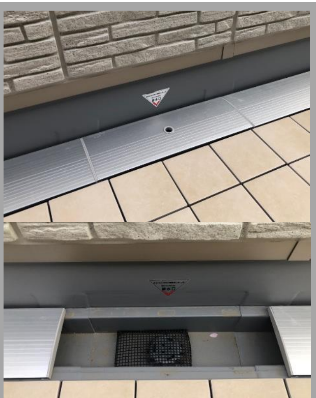
ルーフバルコニー箱樋
