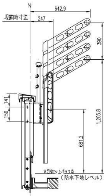
3段手摺タイプ (95mm MI-YR手摺上)
