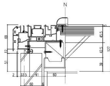
[2 階 FS パルコニー下枠断面]
