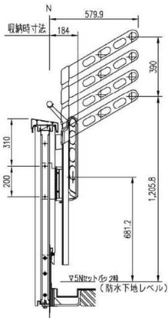
1段手摺タイプ (94mm M-M-YR手摺上)
