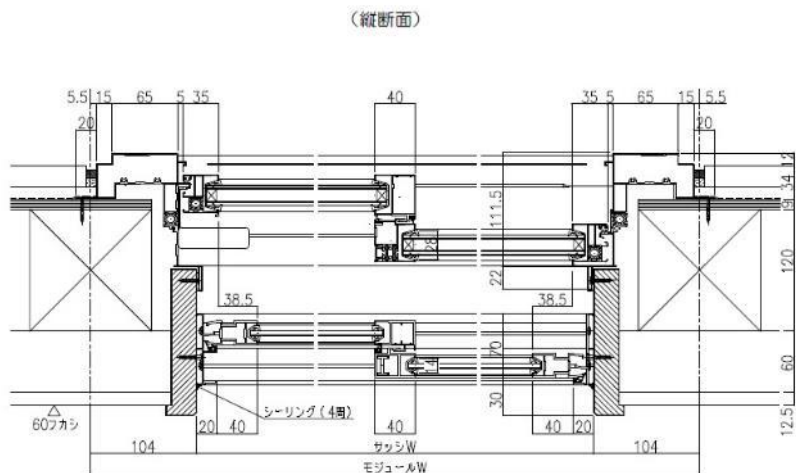
(横断面)
