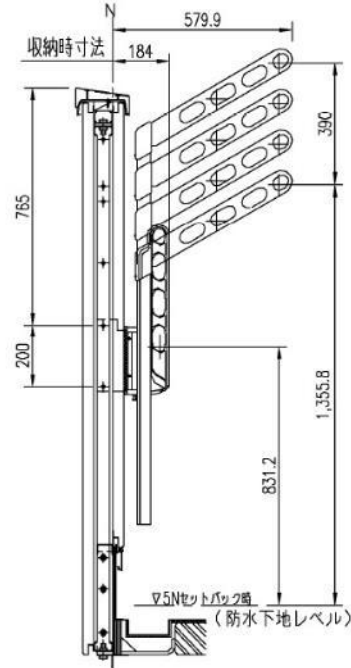
ハイウォールバルコニー
