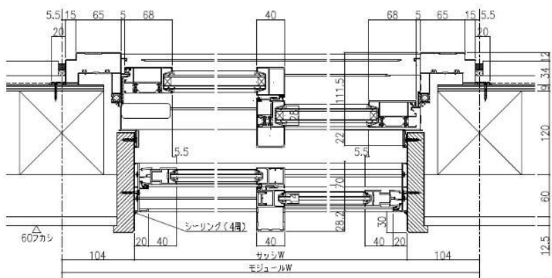
(横断面)
