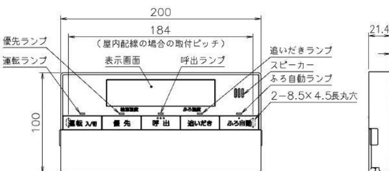
浴室リモコン
