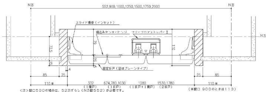
平面詳細図
