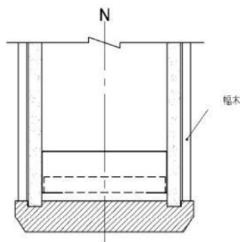
(K2) B-B'断面
