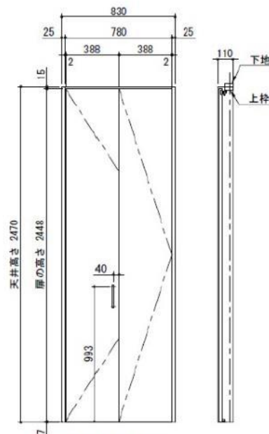
本図は吊元：右を示す
