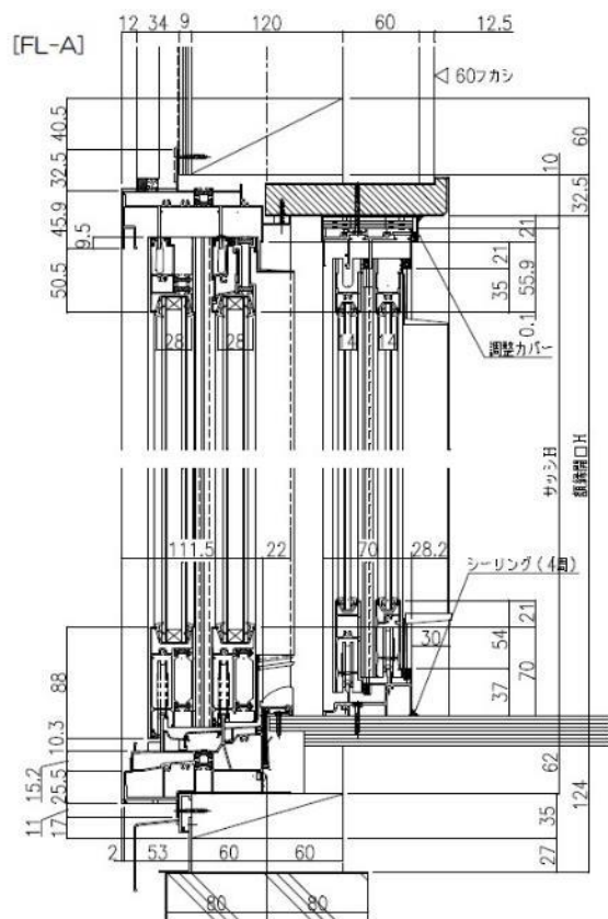
(縦断面)
