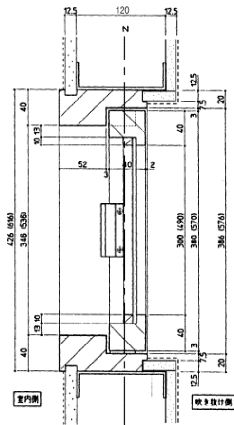
縦断面図
